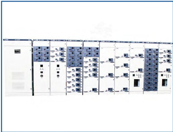
MNS配电柜
